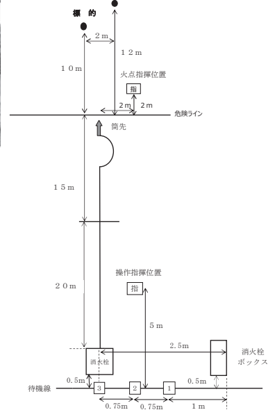
屋外消火栓操法 全体図
